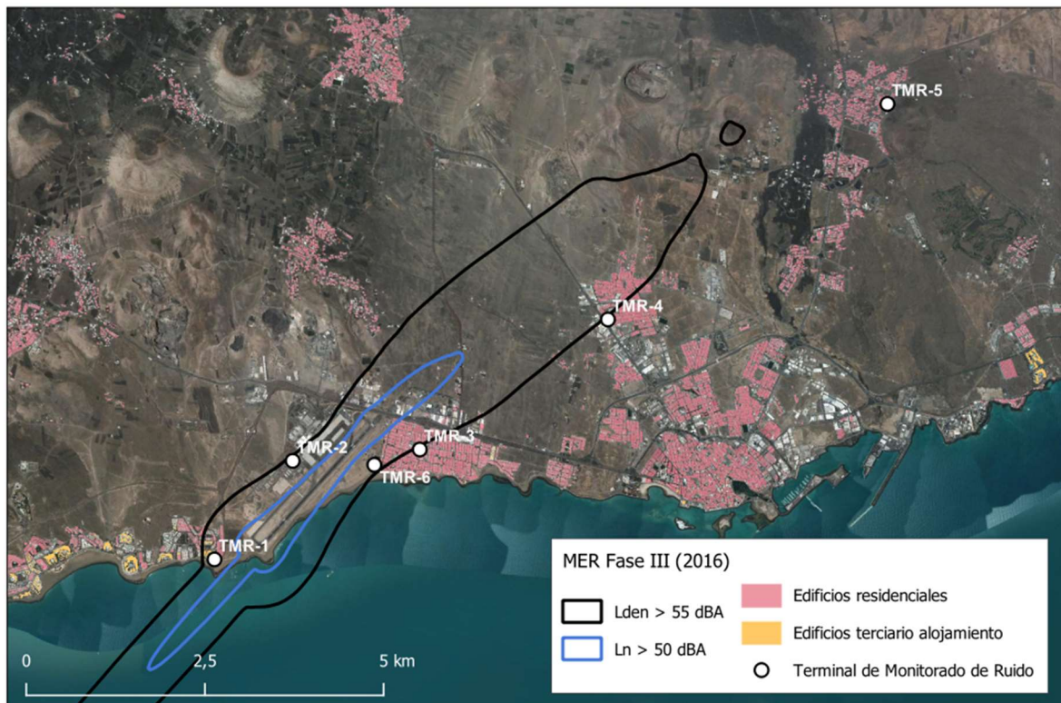
Ilustración 18 Ubicación de los terminales SIRACE. Aeropuerto César Manrique Lanzarote
