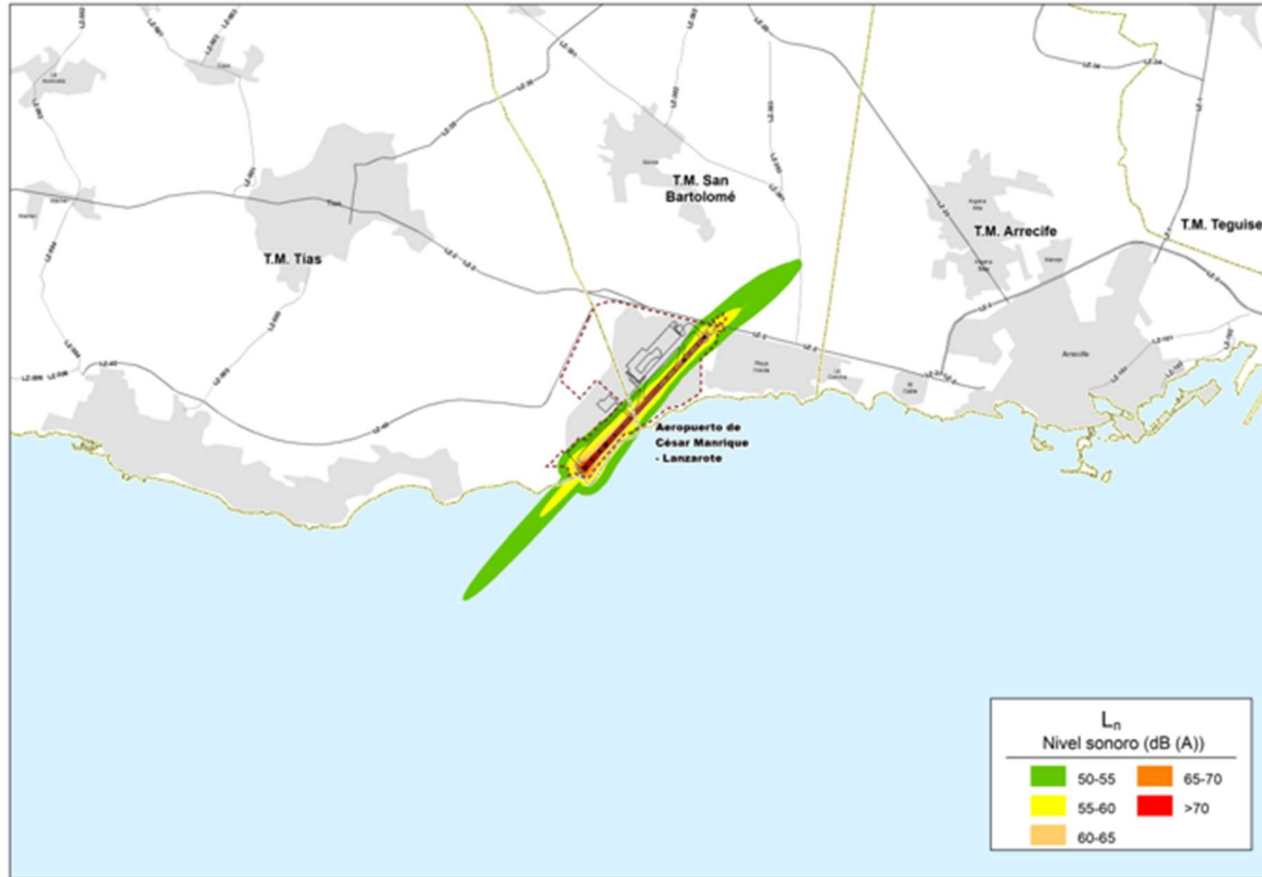
Ilustración 8 Mapa de niveles sonoros Ln. MER Fase III. Aeropuerto César Manrique Lanzarote
