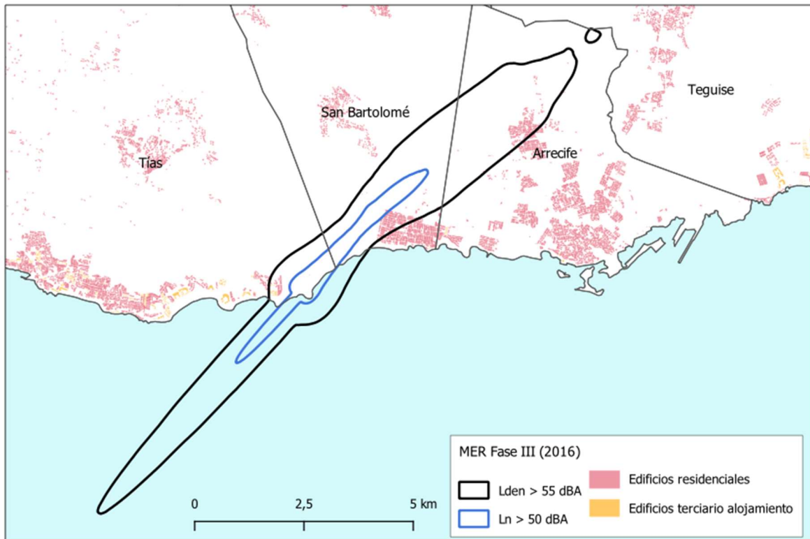
Ilustración 13. Isófonas MER Fase III Aeropuerto César Manrique Lanzarote
