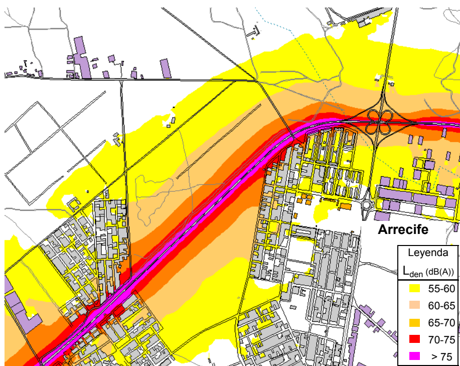
UME-LZ-3: Detalle del mapa de ruido índice L_{den} en Arrecife
