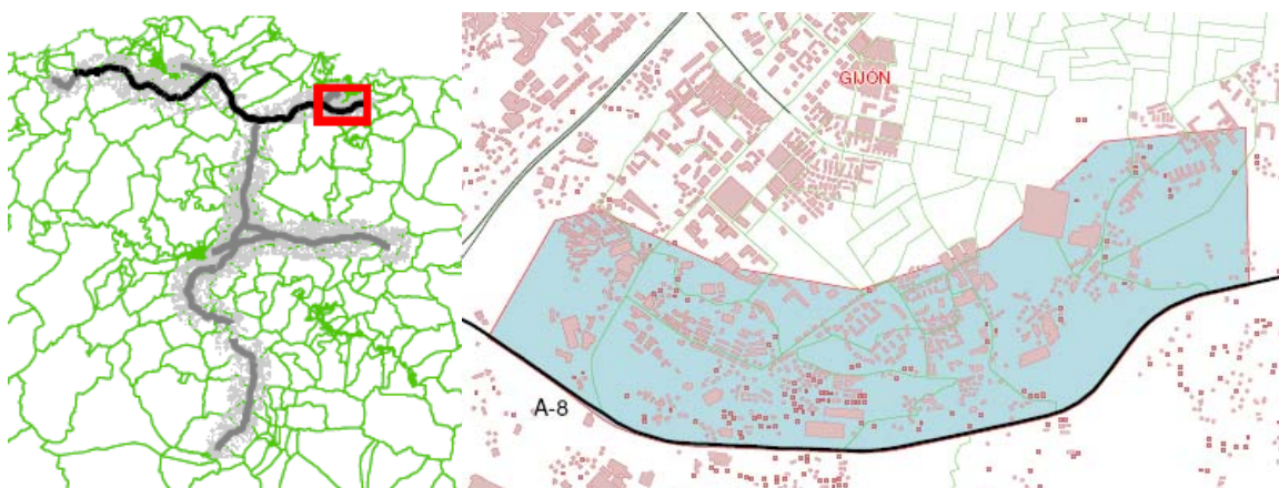
Figura 17. Situación y delimitación de la zona de detalle A-8. Gijón Sur.
