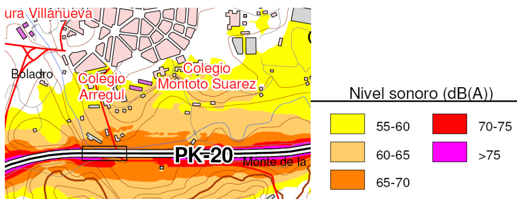
Figura 21. Detalle de niveles acústicos Lden de los colegios.
