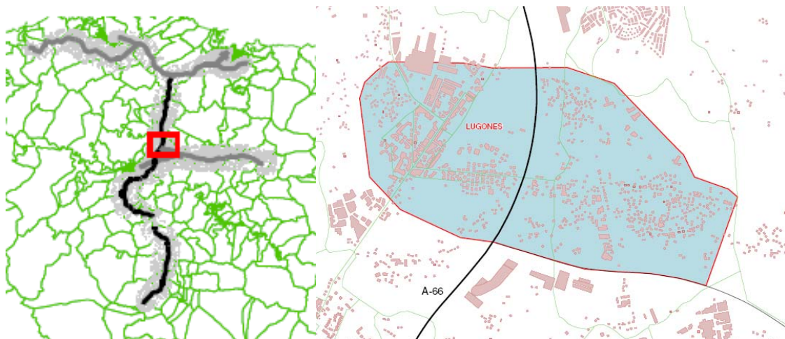
Figura 12. Situación y delimitación de la zona de detalle A-66. Lugones.
