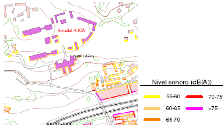
Figura 20. Detalle de niveles de fachada Lden del hospital HUCA.
